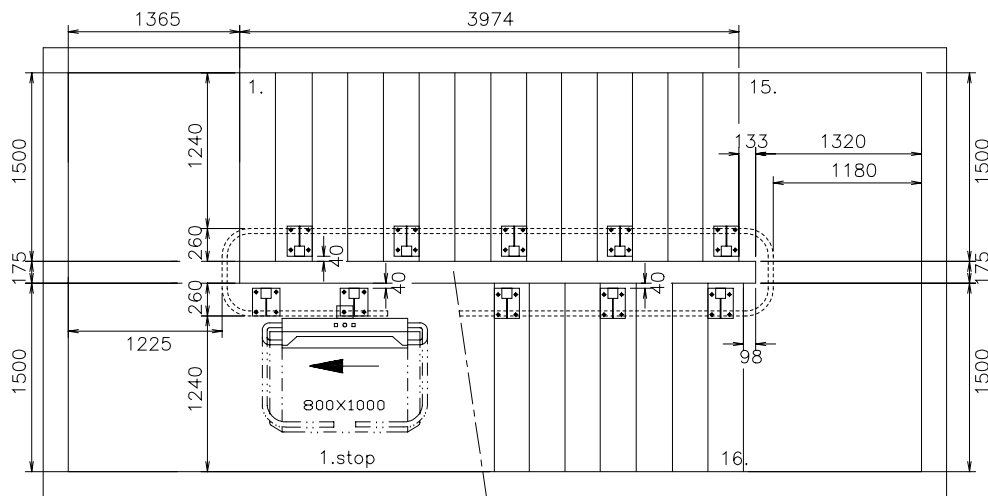
Hélix Fixations par des pieds Escalier tournant
